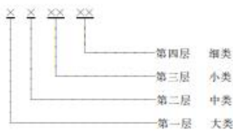
图 1 代码结构
